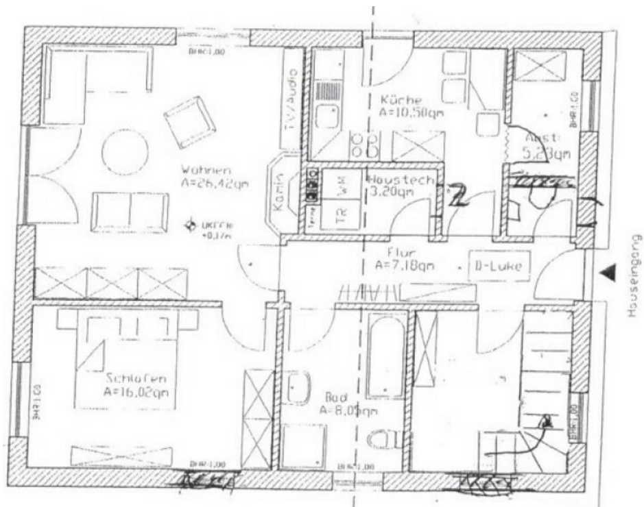
Grundriss EG
