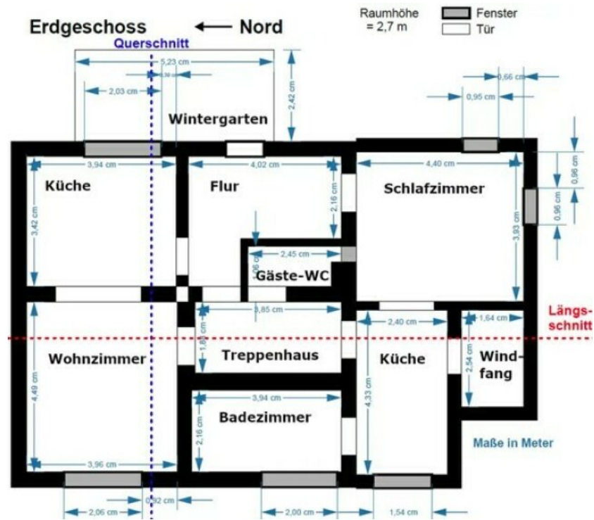
Grundriss EG
