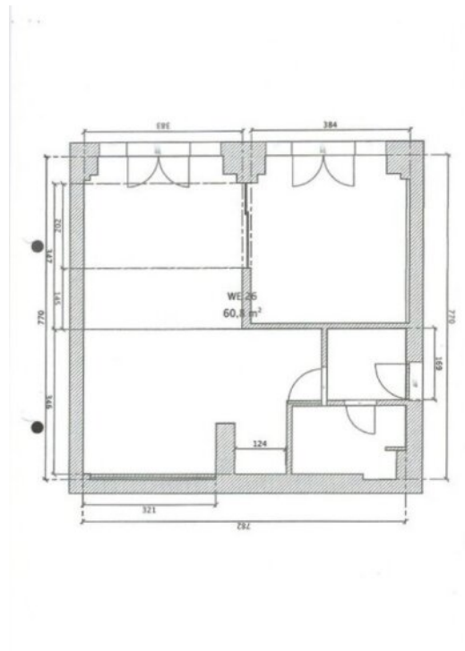
Grundriss
