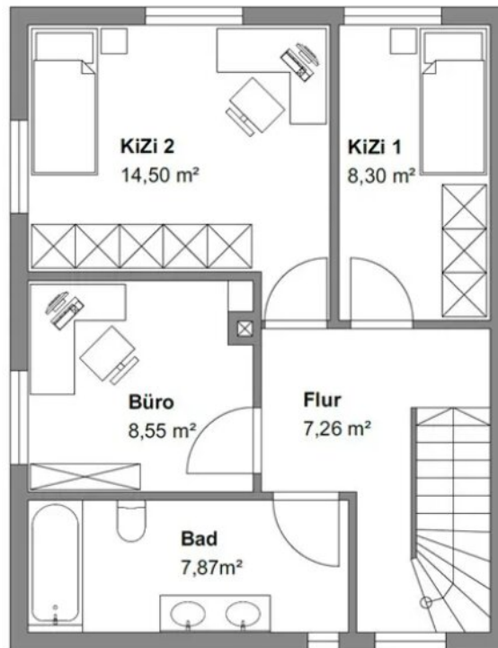
Grundriss OG
