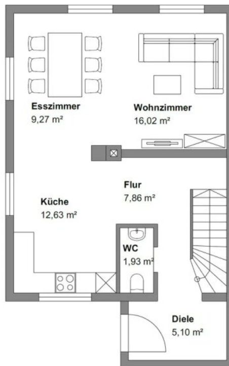
Grundriss EG
