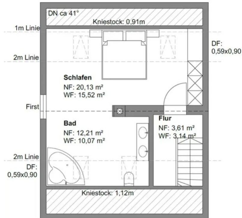
Grundriss DG
