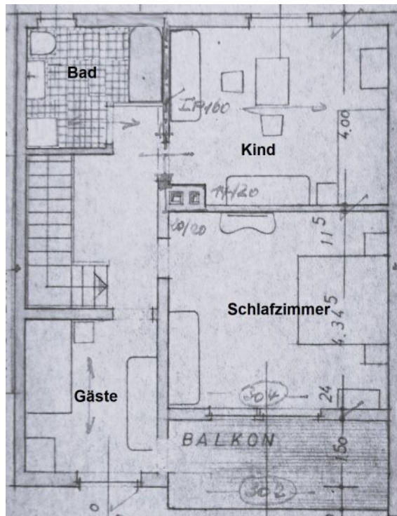
Grundriss OG
