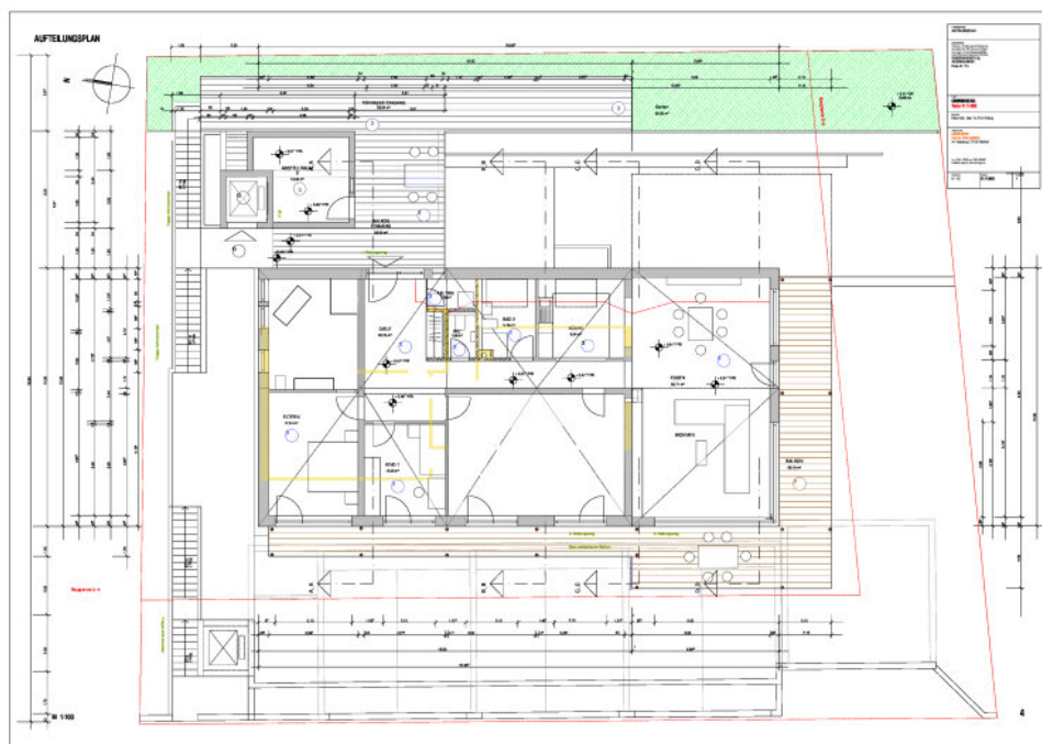
Grundriss-DG
