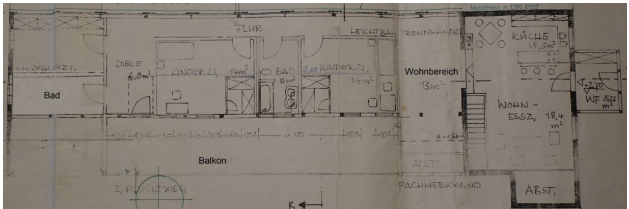
Grundriss
