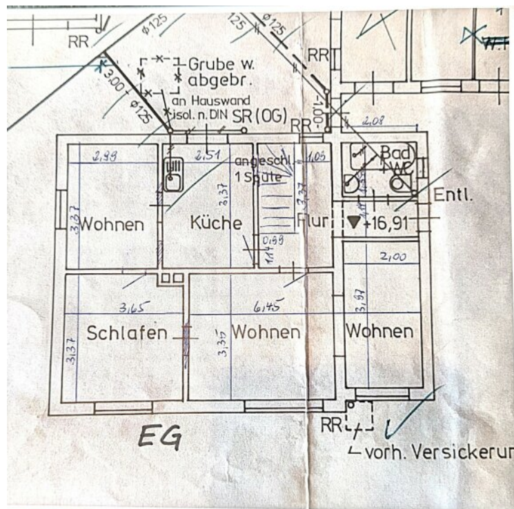
Grundriss Erdgeschoss
