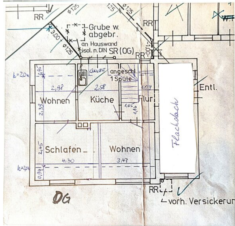
Grundriss Dachgeschoss
