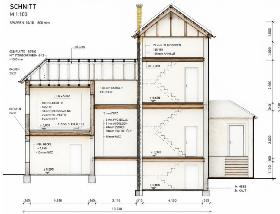
Schnitt
