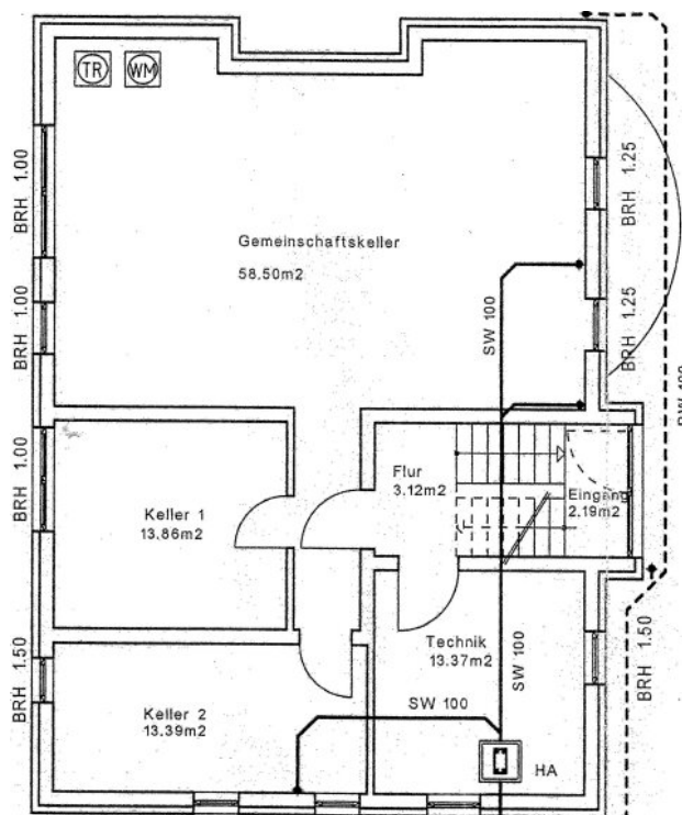
Grundriss Kellergeschoss
