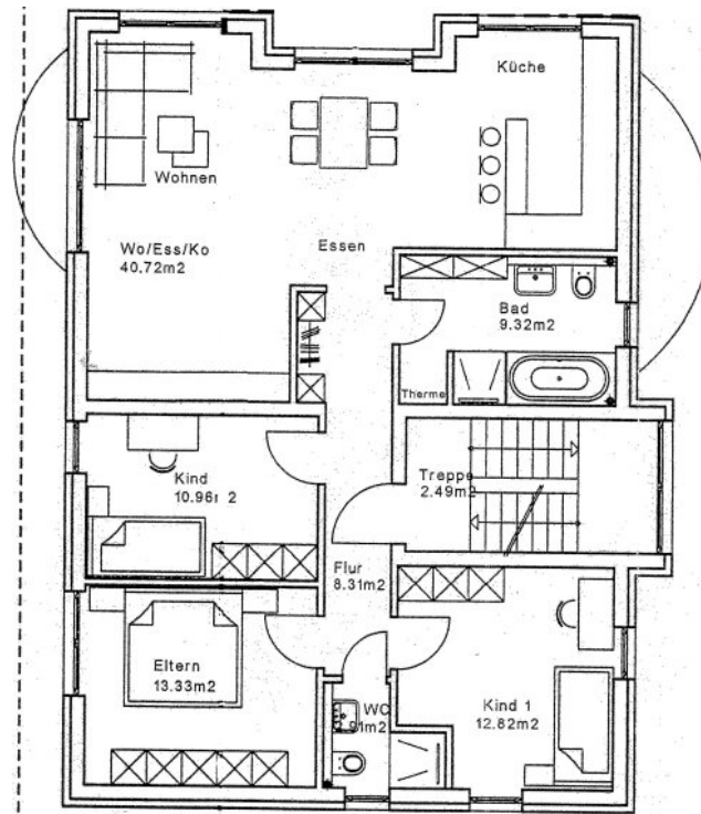
Grundriss Erdgeschoss
