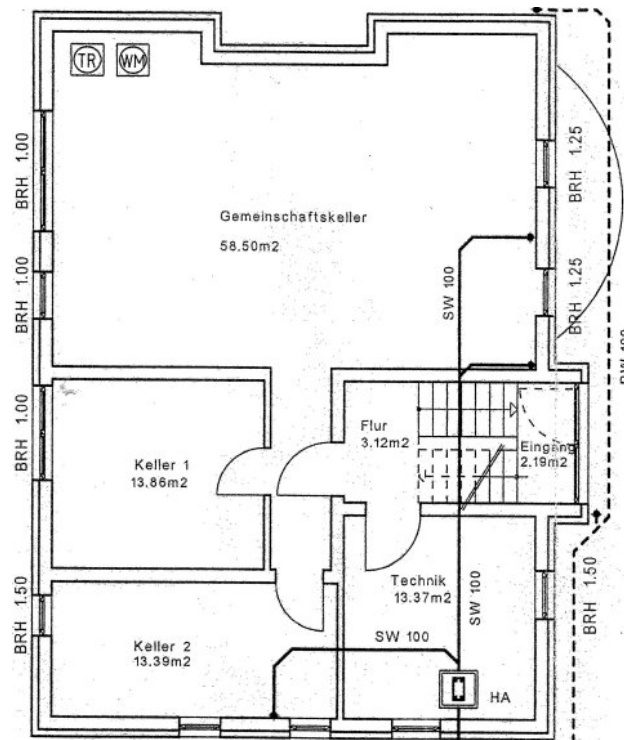
Grundriss Kellergeschoss
