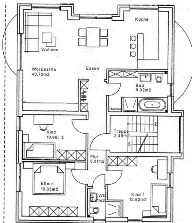
Grundriss Erdgeschoss
