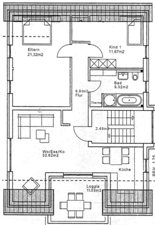
Grundriss Obergeschoss
