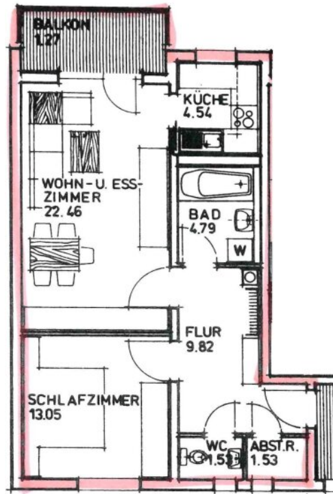
Grundriss
