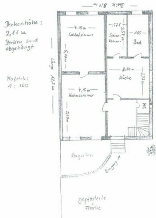
Grundriss EG
