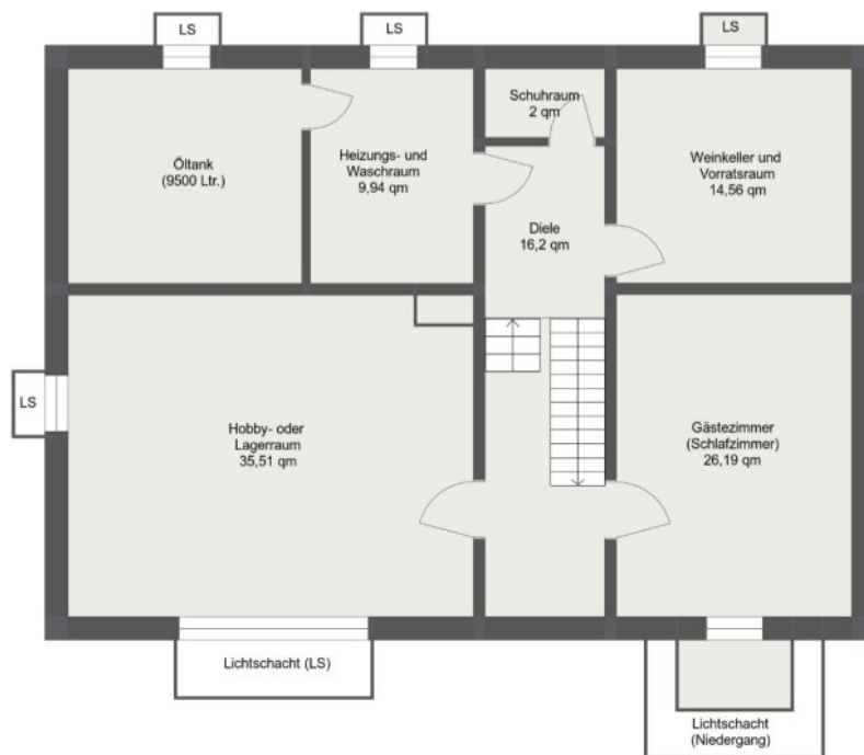
Grundriss UG
