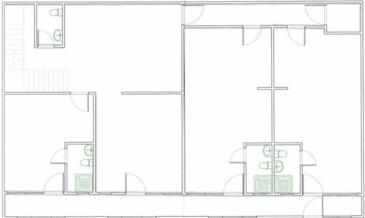
UG Grundriss-Zimmer
