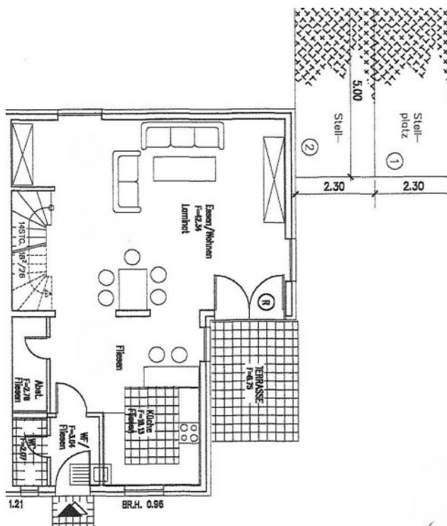
Grundriss EG
