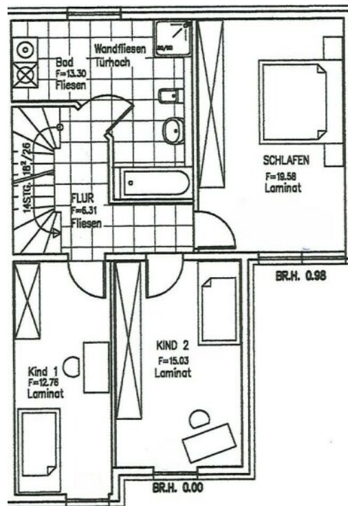
Grundriss OG
