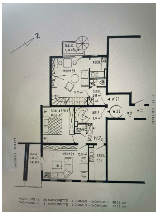
Grundriss UG
