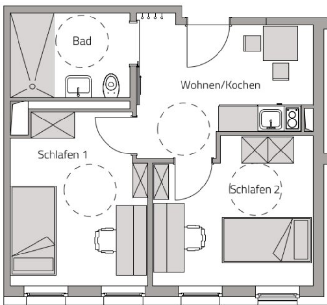
Grundriss
