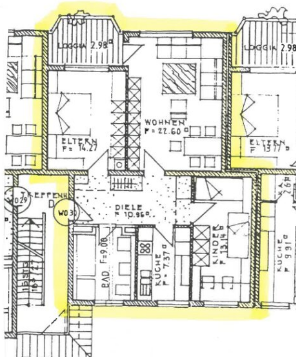
Grundriss
