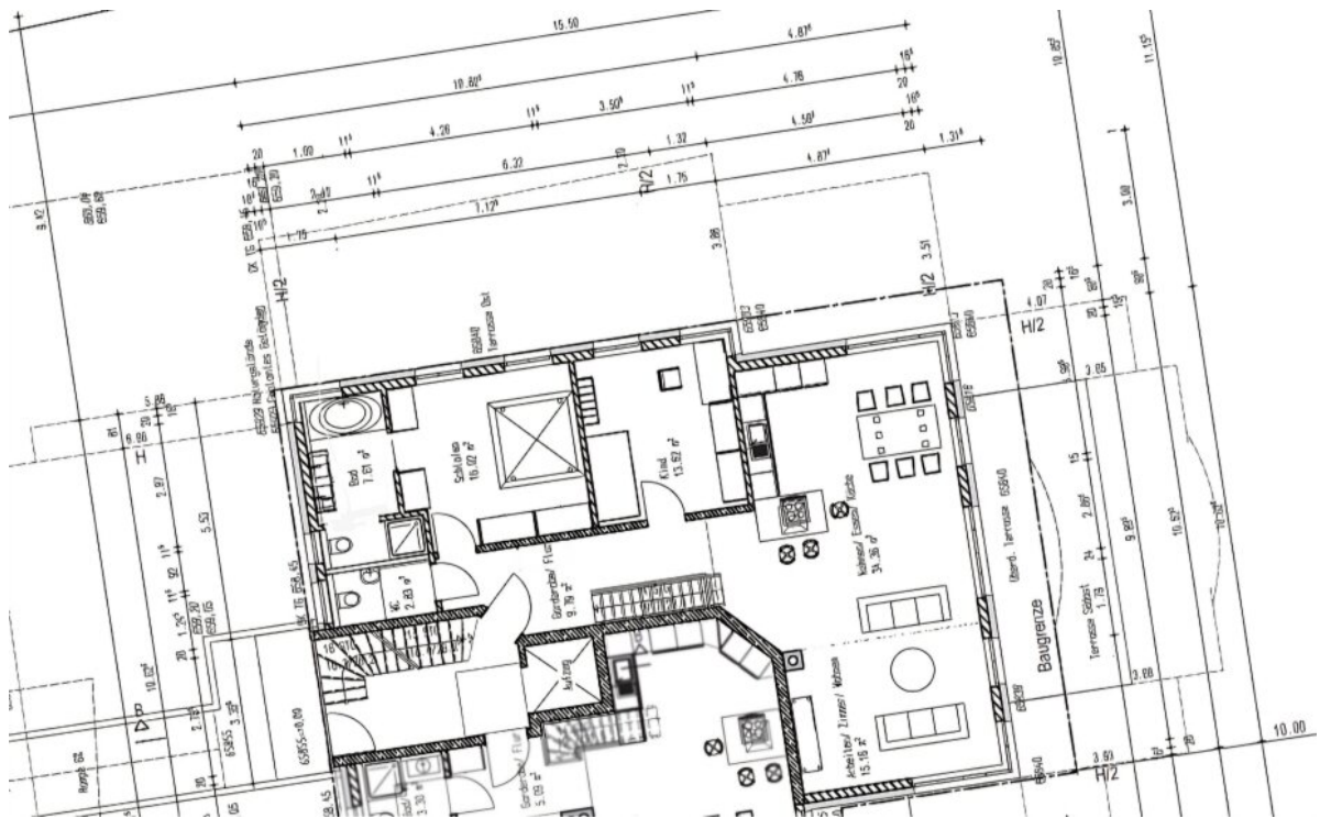
Grundriss EG
