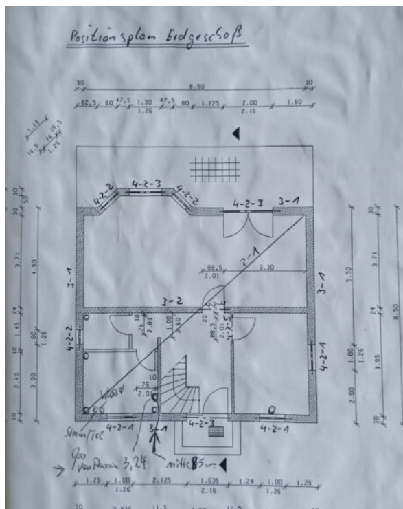
Grundriss Erdgeschoss
