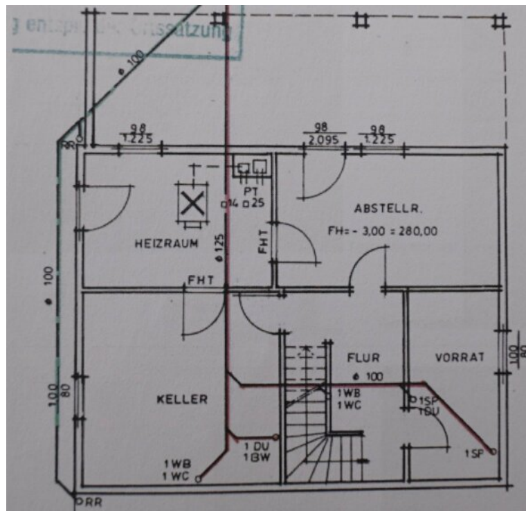
Grundriss KG
