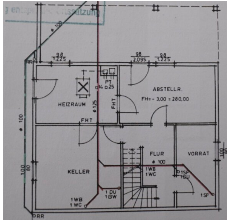
Grundriss KG
