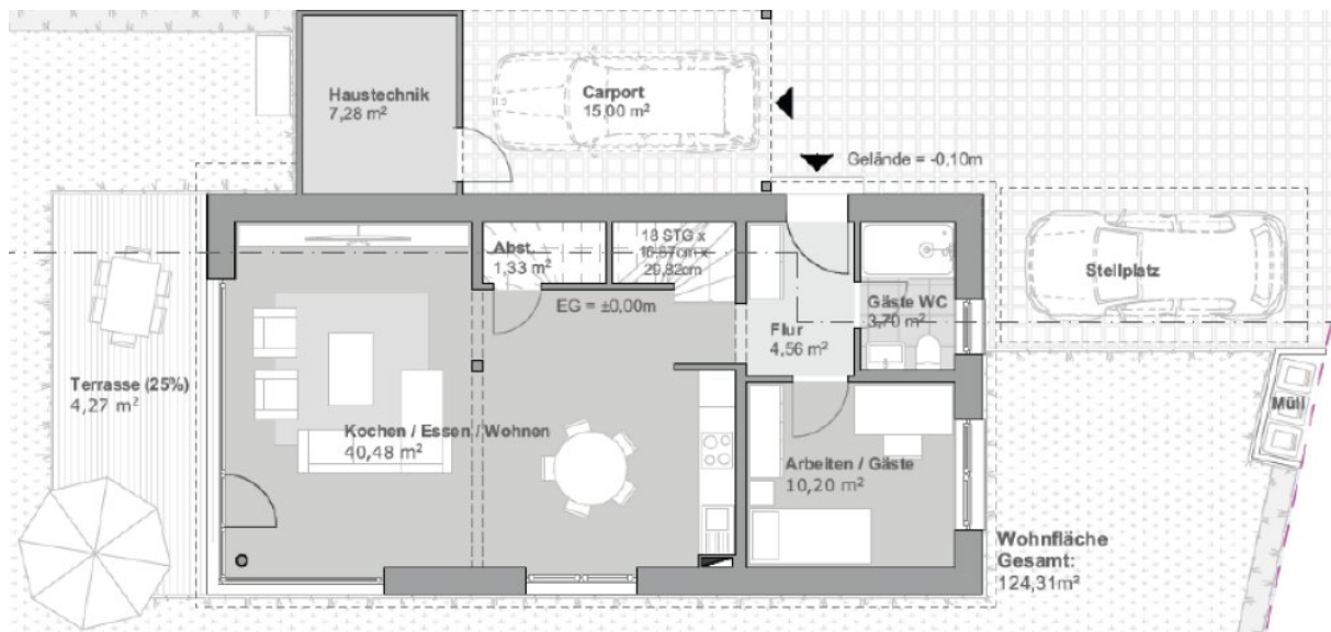
Grundriss EG
