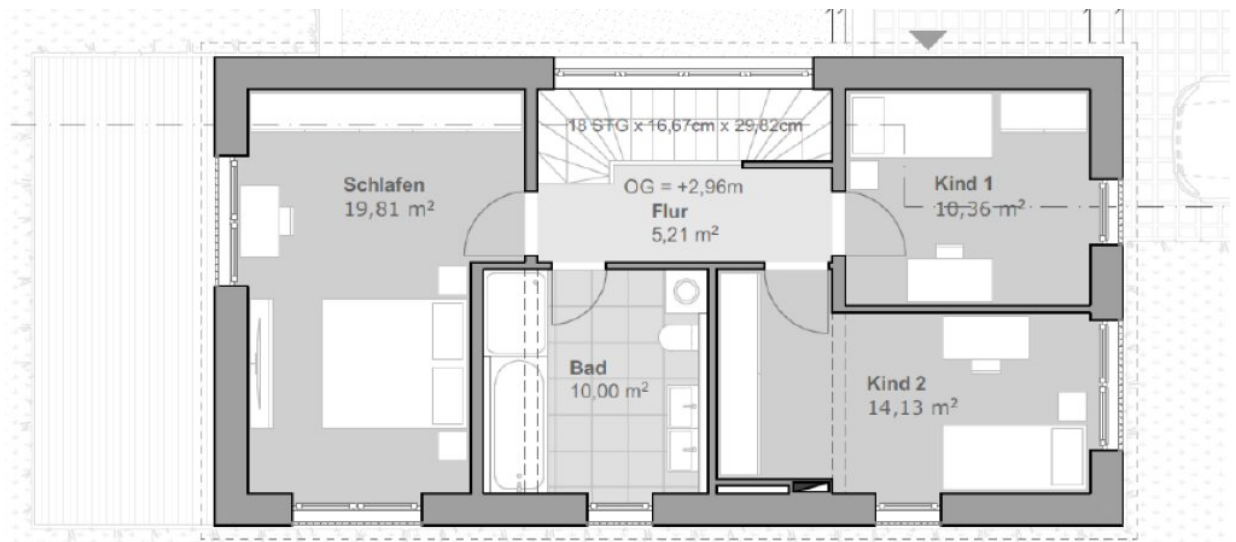
Grundriss OG
