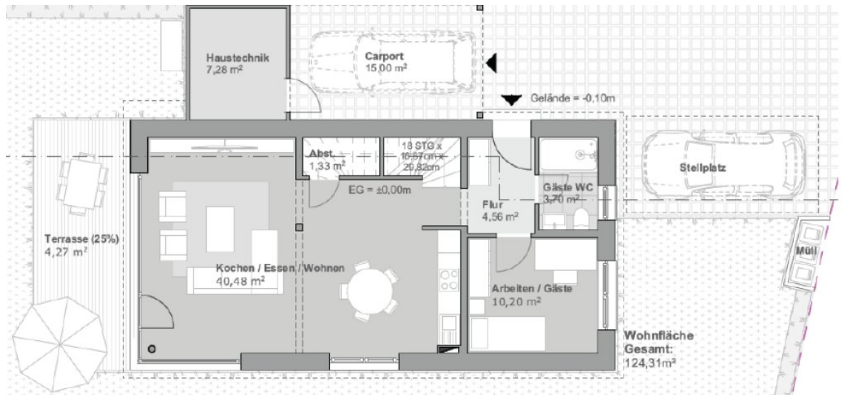
Grundriss EG
