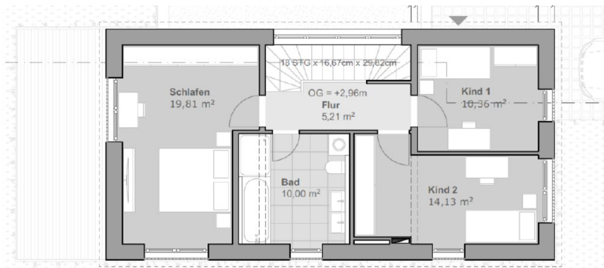
Grundriss OG
