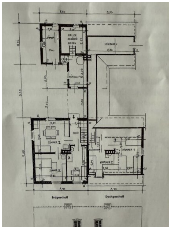
Grundriss
