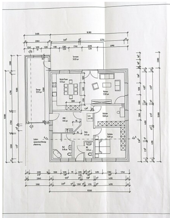
Grundriss
