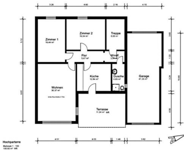
Grundriss Hochparterre
