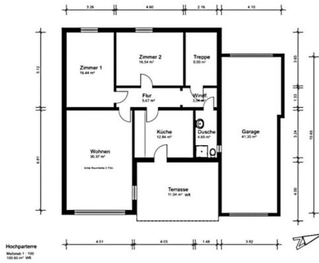
Grundriss Hochparterre
