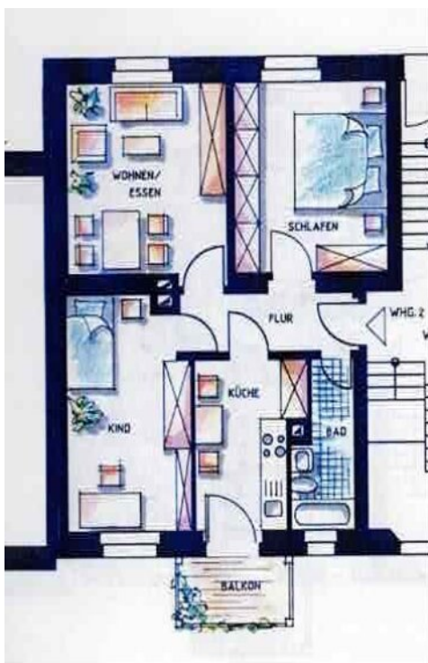
Grundriss
