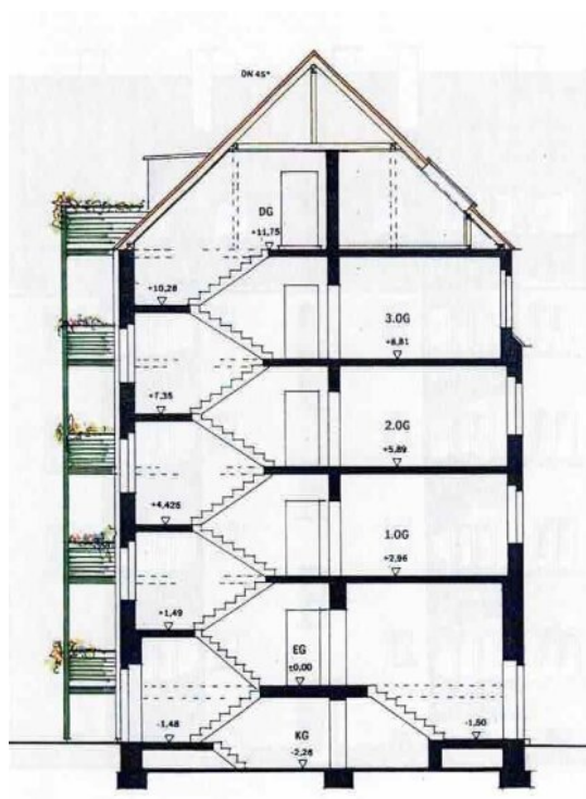
Schnitt
