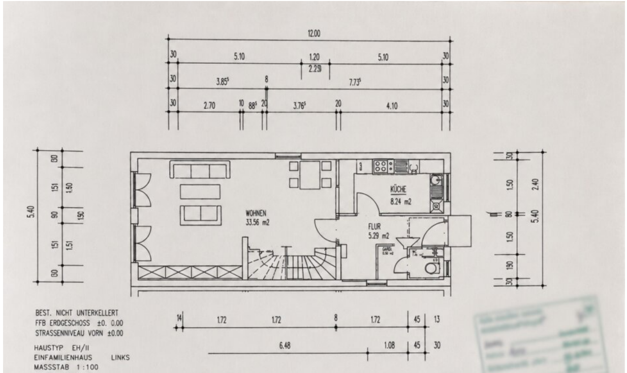
Grundriss EG
