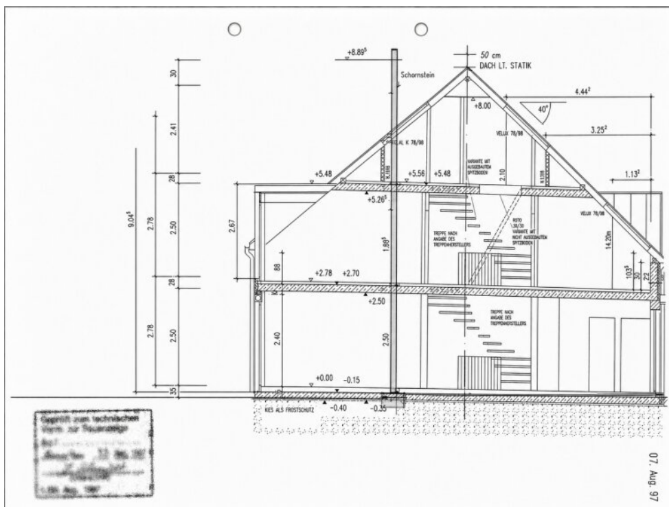
Schnitt Haus
