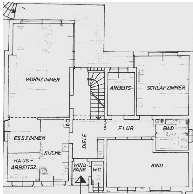
EG Grundriss
