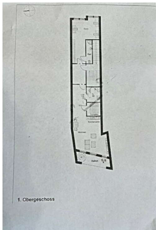
GR 1.OG
