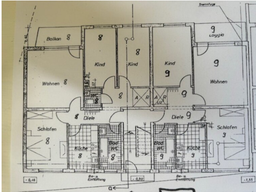
Grundriss
