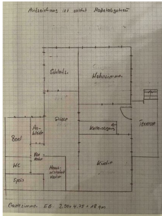
Grundriss EG
