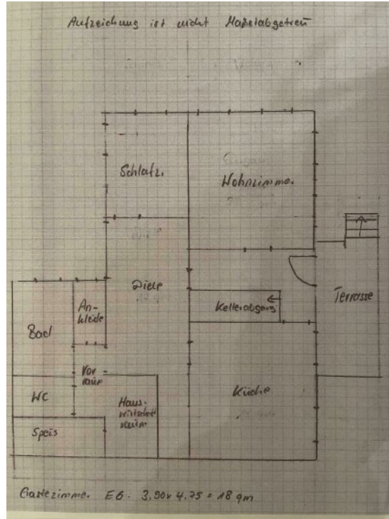
Grundriss EG
