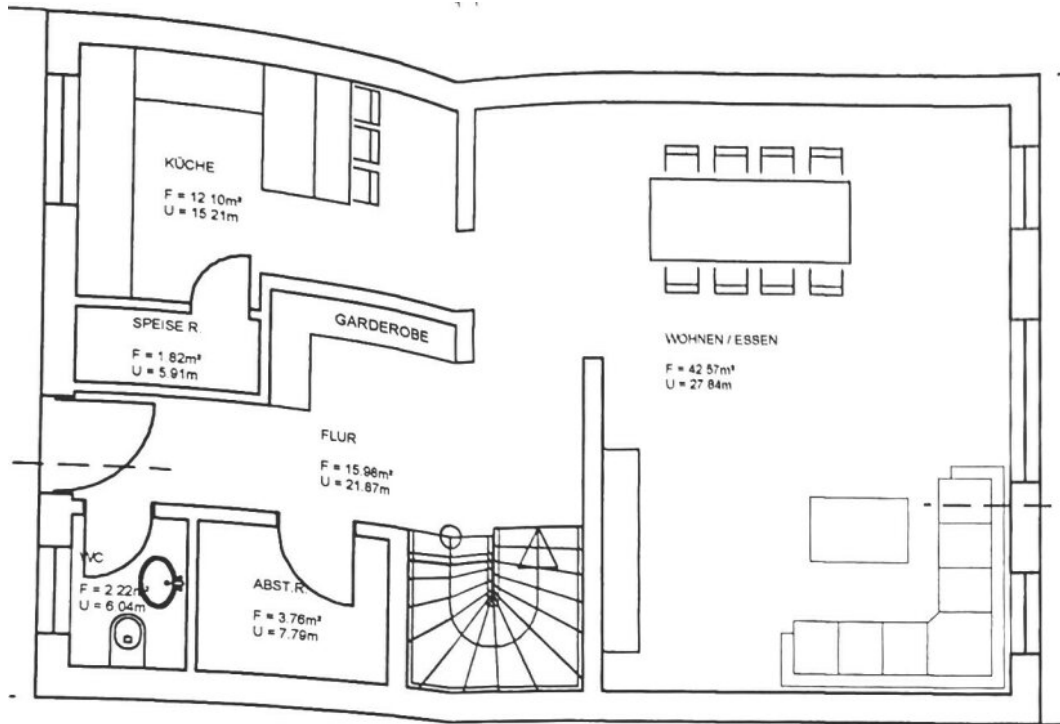
Grundriss EG
