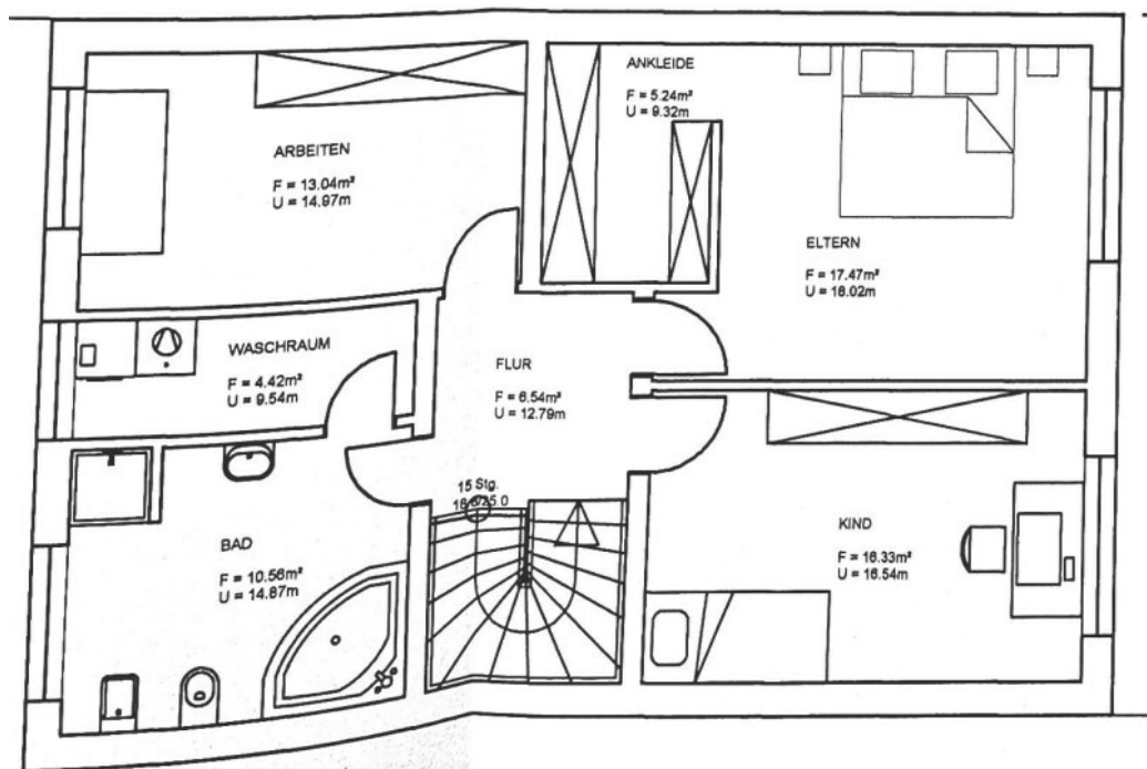
Grundriss OG
