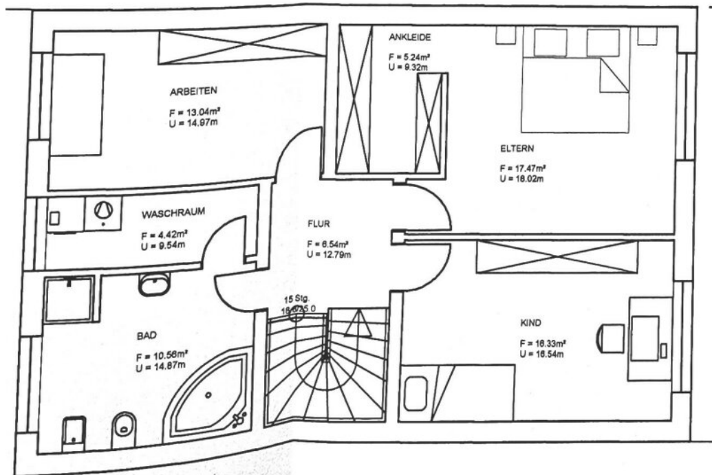
Grundriss OG
