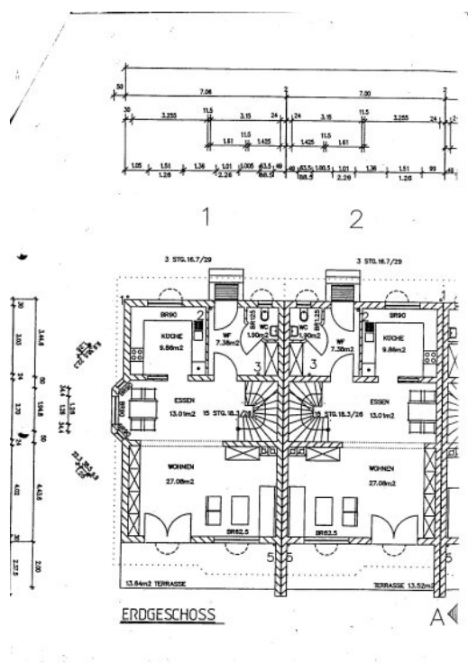
Grundriss Erdgeschoss
