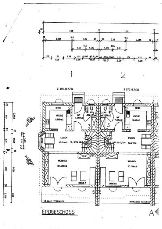
Grundriss Erdgeschoss
