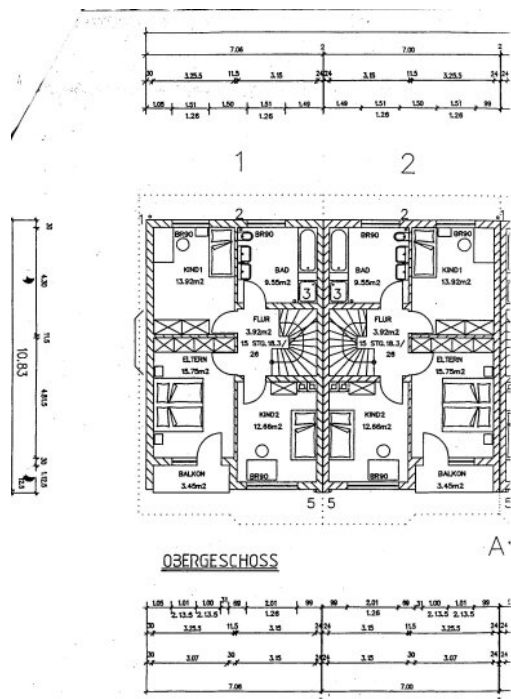
Grundriss Obergeschoss
