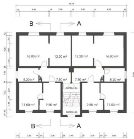
Grundriss: EG, 1.OG, 2.OG
