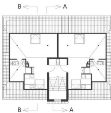
Grundriss: DG
