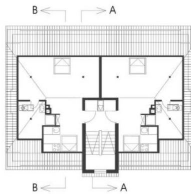
Grundriss: DG
