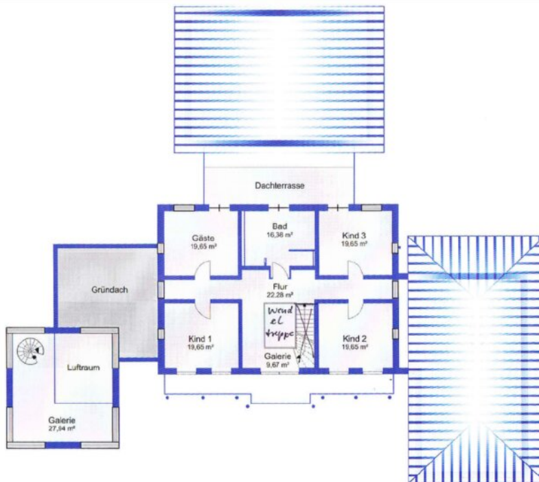
Grundriss OG Wohnhaus
