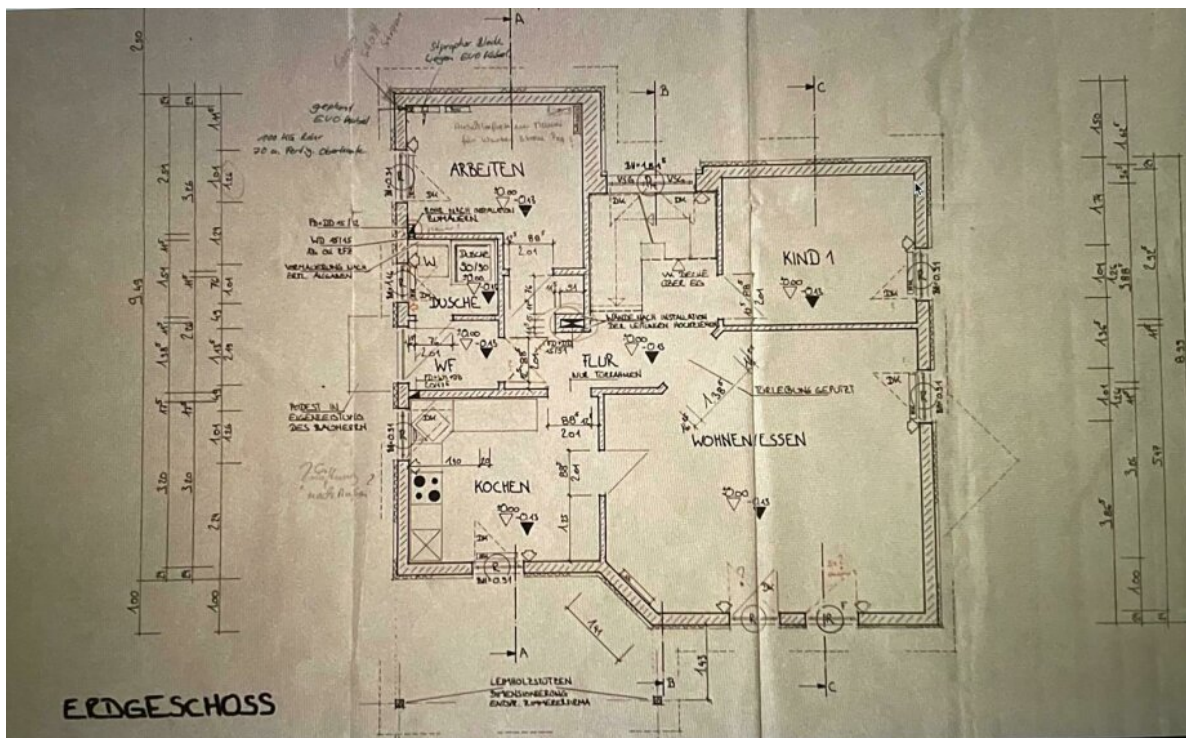
Erdgeschoss
