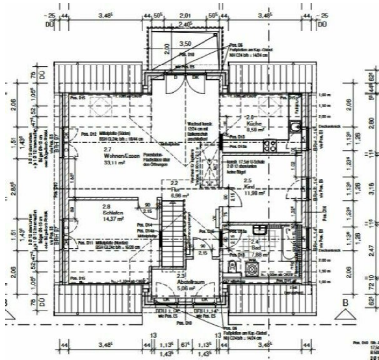
Grundriss EG
