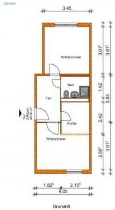
Vermasster Grundriß
