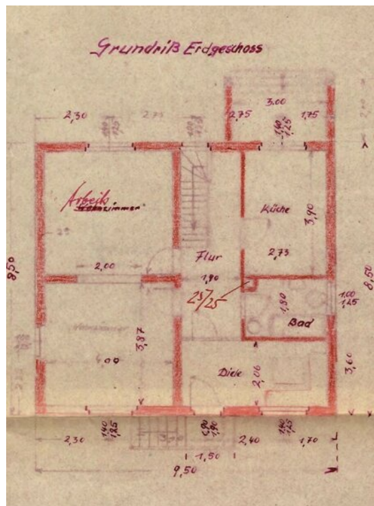
Grundriß Erdgeschoss
