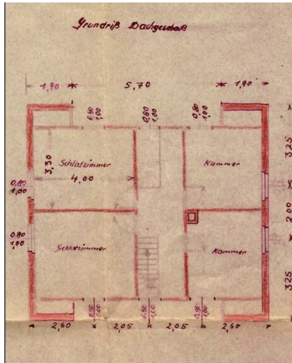
Grundriß Dachgeschoss
