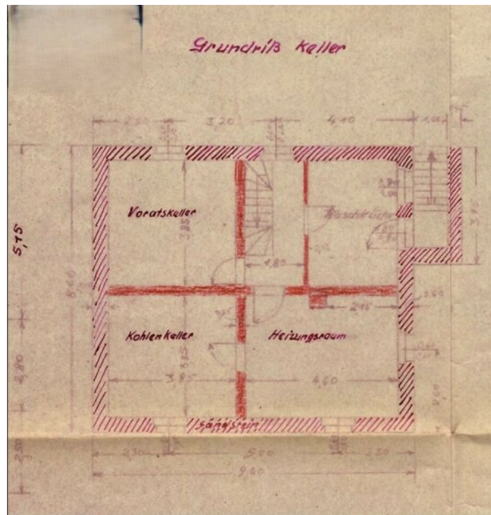
Grundriß Kellergeschoss
