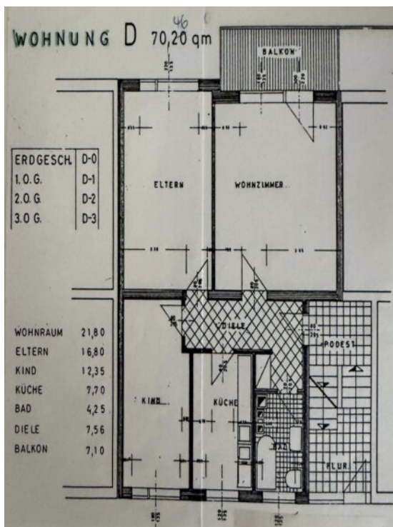
Grundriss
