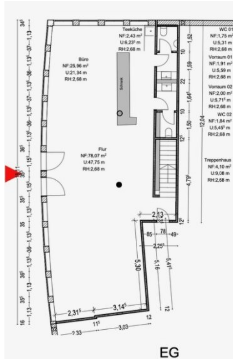
Grundriß EG
