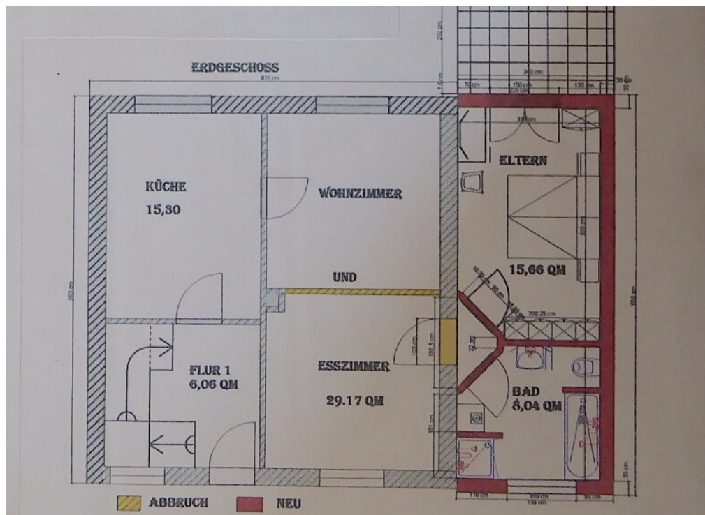
Grundriss EG
