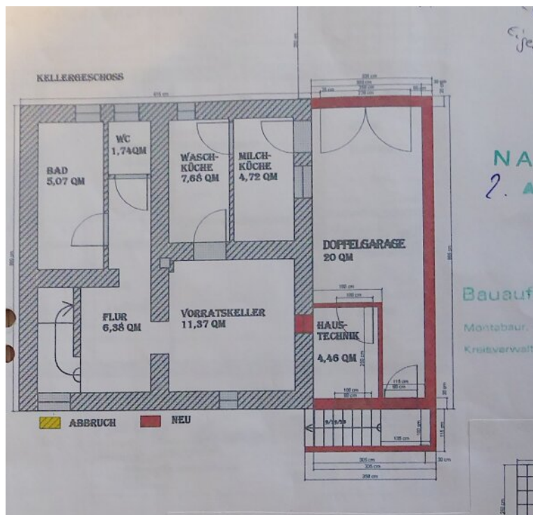
Grundriss Keller
