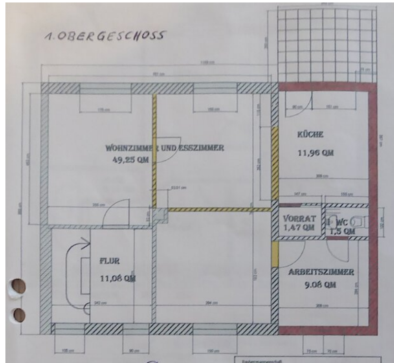
Grundriss OG
