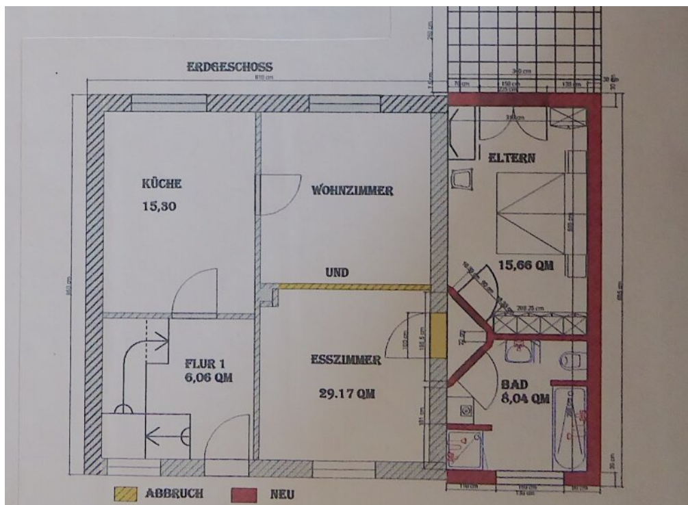
Grundriss EG
