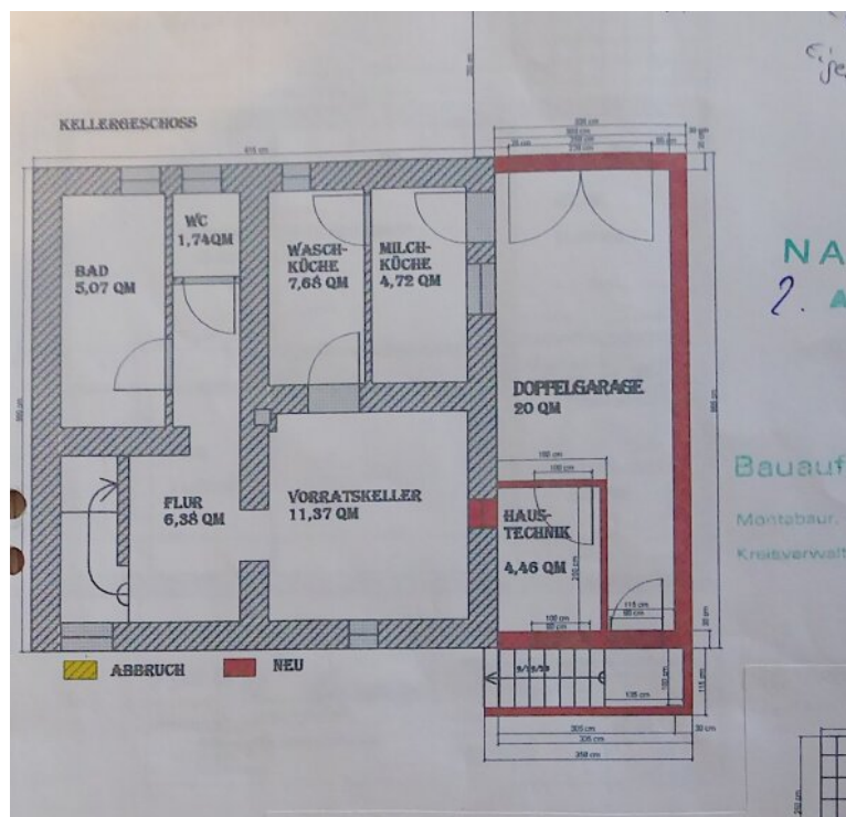
Grundriss Keller
