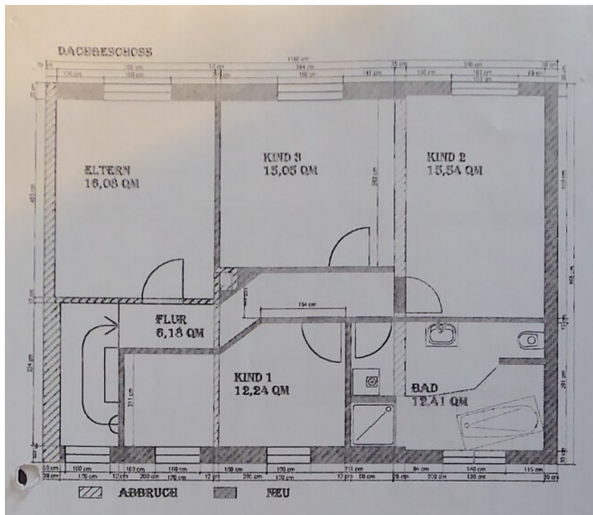
Grundriss DG
