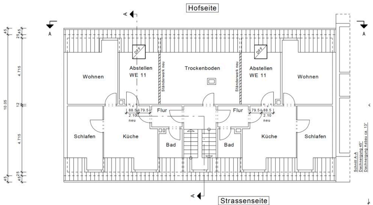
Grundriss - DG
