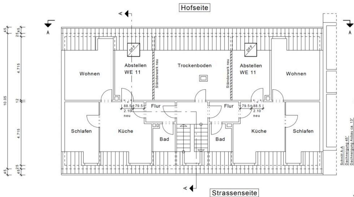
Grundriss - DG
