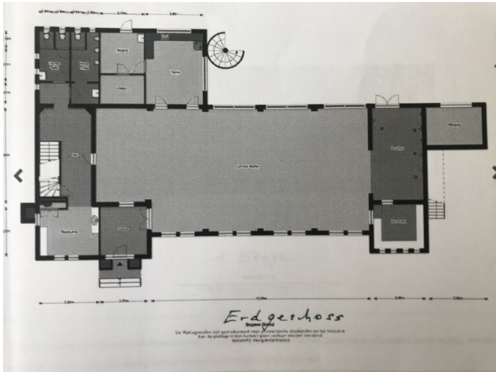
Grundriss EG
