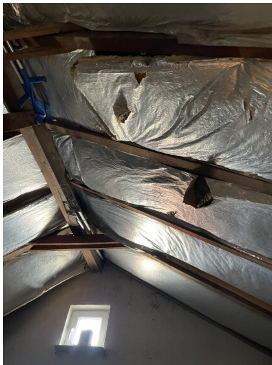
Dachstuhl isoliert
