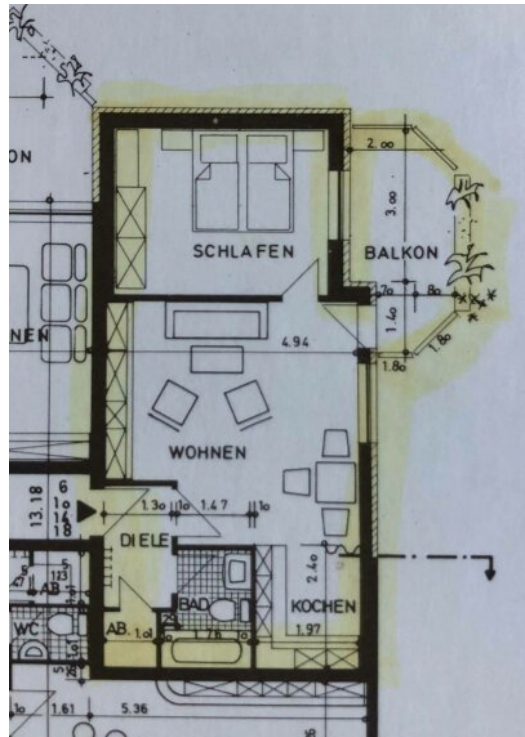
Grundriss
