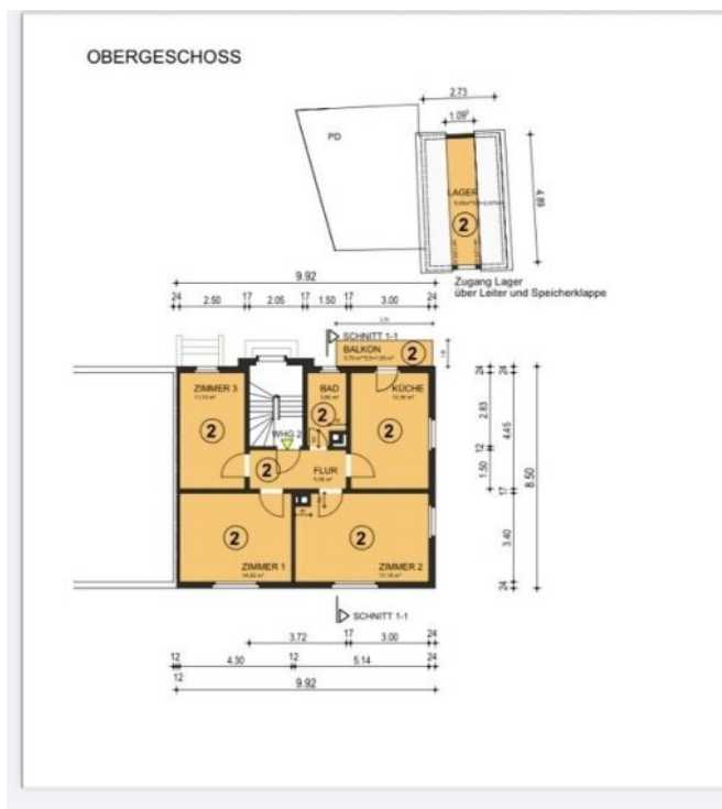
OG-Grundriss
