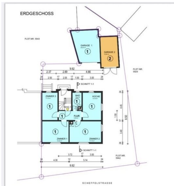
EG-Grundriss
