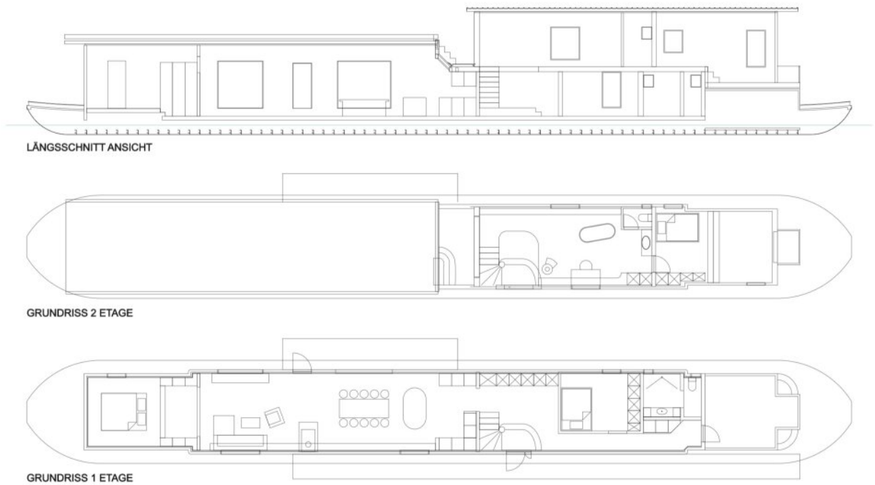
Geplante Grundrisse
